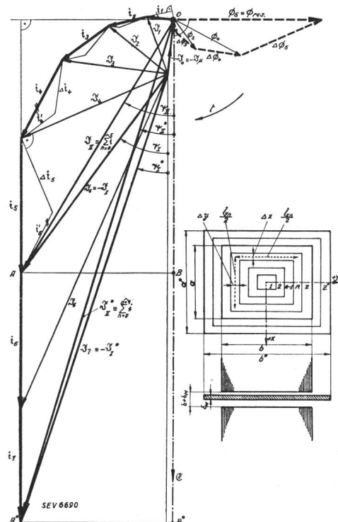
Fig. 9. Spiraldiagramm für Zonenstrom und Zonenfluss, dargestellt am Beispiel einer rechteckigen Kupferplatte im Luftspalt eines Eisenkerns, die von einem 50periodigen Wechselfluss durchsetzt wird. Luftspalt \delta = 0 , Plattenstärke \delta_M = 0,1 \text{ cm} , B_0 = 1000 \text{ Gauss} .
