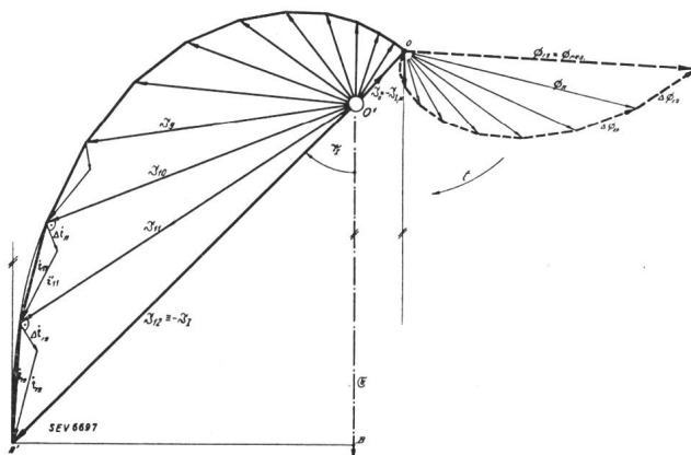
Fig. 12. Spiraldiagramm für den Kupferzylinder eines nutenlosen Rotors.
