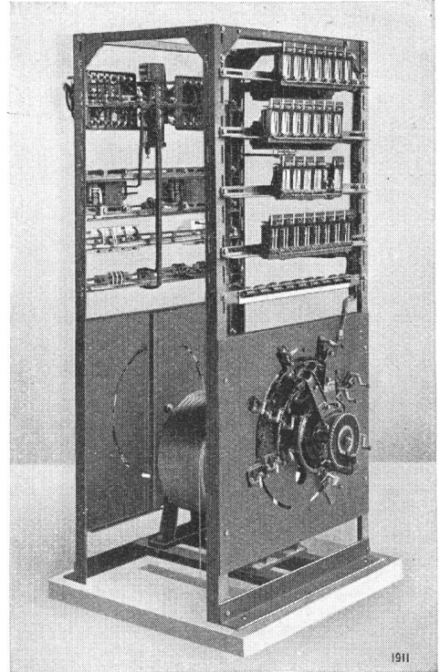
Kollektiv-Selektiv-Steuerung für Personenaufzüge, der Firma Schindler & Cie. A.-G.
