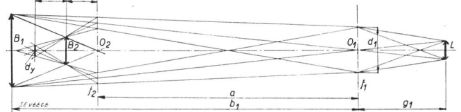
Fig. 2. Strahlengang.
