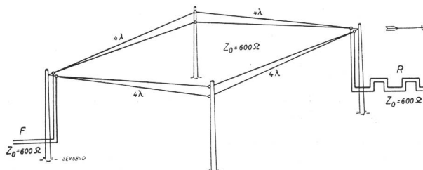
Fig. 6. Antenne rhombique. R Résistance d'extrémité. F Ligne d'alimentation.
