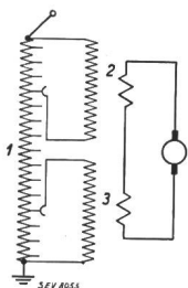
Fig. 3. Schaltprinzip der Hochspannungssteuerung. 1 ein Transformator mit Anzapfungen. 2, 3 zwei gleiche Transformatoren ohne Anzapfungen auf gemeinsamem Eisenstell.
