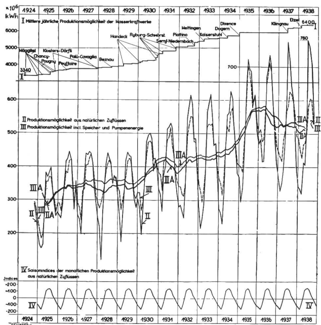
Fig. 1. Energiedarbietung der schweizerischen Elektrizitätswerke von 1924 bis 1938.
