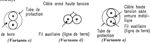
Fig. 1. Mise-à-terre par le neutre.
