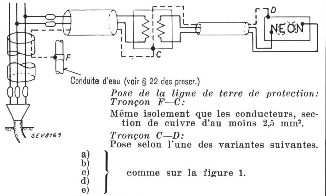
Fig. 3. Mise-à-terre de protection.
