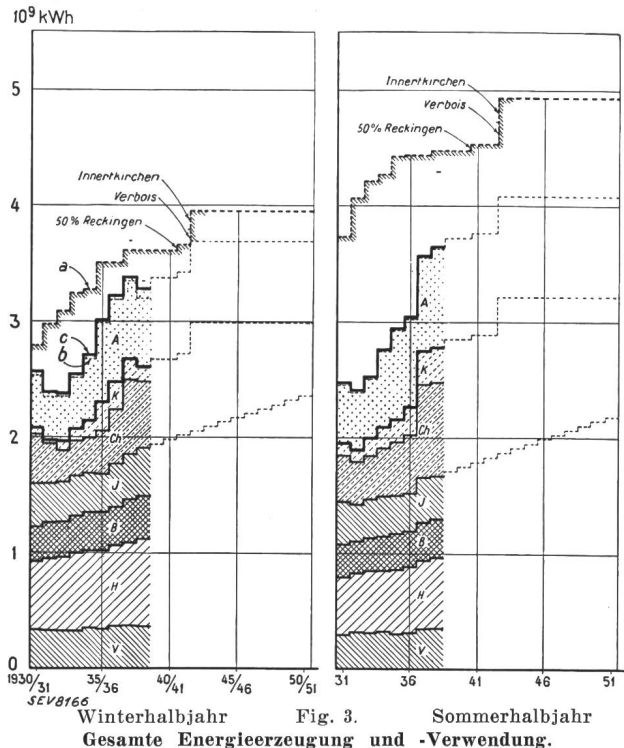
Fig. 3. Gesamte Energieerzeugung und -Verwendung. a Mittlere Produktionsmöglichkeit der Wasserkraftwerke. b Wirkliche Produktion der Wasserkraftwerke. c Gesamtproduktion (inkl. thermische Erzeugung und Einfuhr). Energieverwendung. V Uebertragungsverluste. Ch Elektrochem., -metall. u. -therm. Anwendungen. H Haushalt und Gewerbe. B Bahnen. K Elektrokessel. J Allgemeine Industrie. A Ausfuhr.
