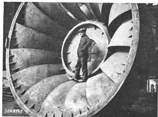
Fig. 4. Lauftrad für das Kraftwerk Sungari (unverputzt). (Escher-Wyss.)
