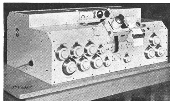
Fig. 2. Rechenggerät für die Fliegerabwehrartillerie.
