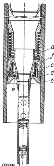
Fig. 15 Düsenschnellkontakt.
