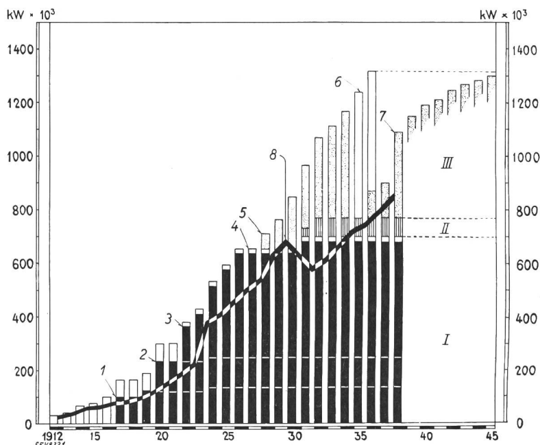
Fig. 3. Développement des puissances disponibles (colonnes) et des puissances maxima (courbe) dans le réseau du Niagara de l'Hydro.
