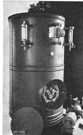
Fig. 2. Akkumulierdampfkessel.
