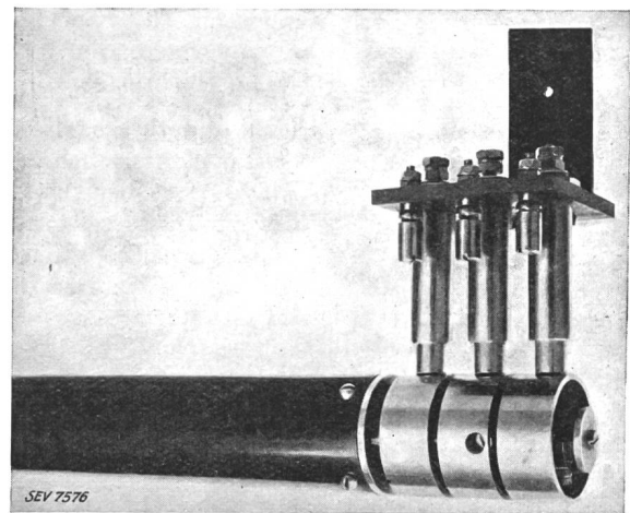
Fig. 3. Walzenheizung, 4 kW, zum Einschleiben in Trockenzyylinder.
