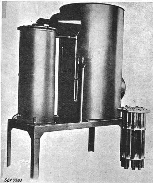
Fig. 10. Destillierapparat 50 kW.
