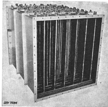
Fig. 13. Lufterhitzer, 100 kW.
