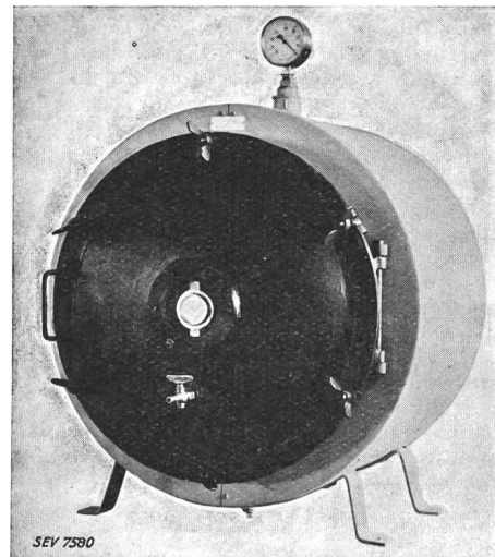
Fig. 7. Laboratoriums-Vakuumschrank.
