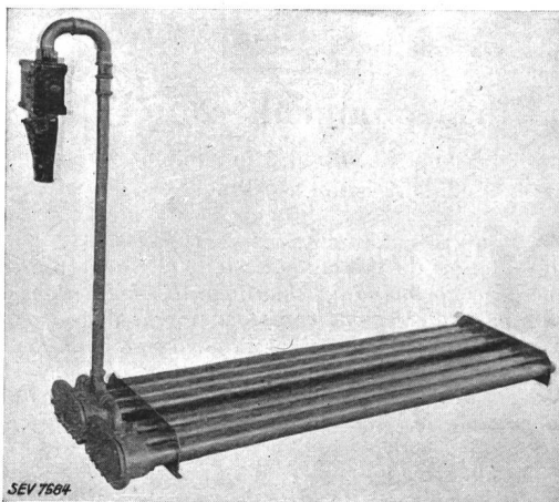
Fig. 11. Tauchheizkörper 30 kW.
