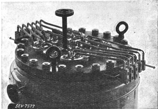
Fig. 4. Ölheizkessel (Anschlüsse).
