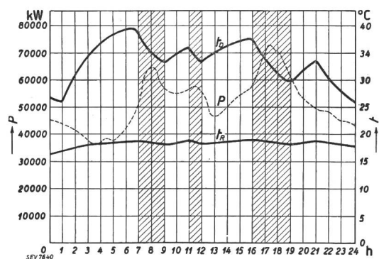
Fig. 4. Deckenheizung. Temperaturverlauf bei den schraffierten Sperrzeiten: t 0 an den Deckenoberflächen und t R im Raum. P Wintertagbelastungsdiagramm des EW Zürich.
