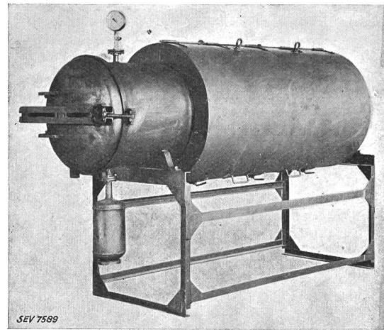
Fig. 16. Vakuumpessel.
