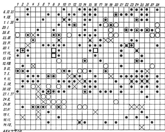
Fig. 1. Perioden-Tafel.
