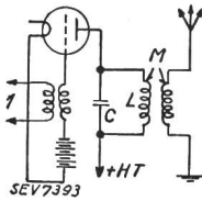
Fig. 3 (en haut). Dernier étage d'amplification.
