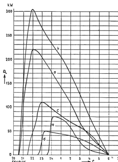
Fig. 3. Mittlerer Belastungsverlauf von Heisswasserspeichern. a 486 Kleinspeicher, Einschaltz. ca. 21 Uhr. b 361 Grosspeicher, Einschaltz. ca. 21 Uhr. c 54 Grosspeicher, Einschaltz. ca. 22 Uhr. d 31 Grosspeicher, Einschaltz. ca. 23 Uhr. e 64 Grosspeicher, Einschaltz. ca. 24 Uhr.
