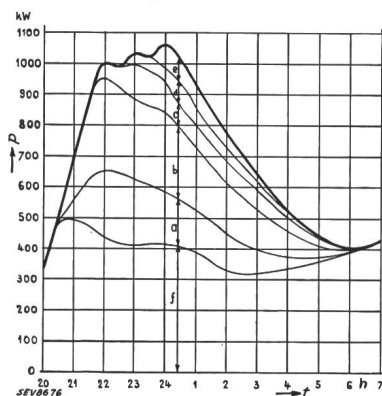
Fig. 4. Belastungsverteilung auf der untersuchten Leitung in einer mitt- leren Sommernacht. a 486 Kleinspeicher, Einschaltz. ca. 21 Uhr. b 361 Grosspeicher, Einschaltz. ca. 21 Uhr. c 54 Grosspeicher, Einschaltz. ca. 22 Uhr. d 31 Grosspeicher, Einschaltz. ca. 23 Uhr. e 64 Grosspeicher, Einschaltz. ca. 24 Uhr. f Grundlast.
