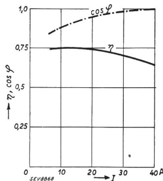
Verlauf von Wirkungsgrad und Leistungsfaktor \cos \varphi in Funktion des Ladestromes I einer Batterie von 20 Pb-Zellen.
