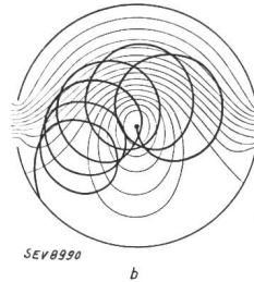
Fig. 6. Aequipotentiallinien und Elektronenbahn in einer Magnetfeldröhre nach Fig. 5. a Vereinfachtes Schema mit ebenen Elektroden. b Die wirkliche Magnetfeldröhre.
