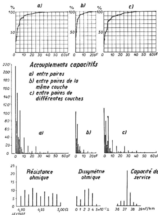
Fig. 4. Câble téléphonique, 40 paires 1,3 mm \varnothing , conducteurs en aluminium. Abscisses: valeurs mesurées. Ordonnées: nombres de valeurs correspondantes.
