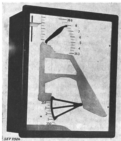
Fig. 4. Stellungsfernzeiger einer Wehrklappe und eines Schiebers in der Zuleitung zu einer Turbine.
