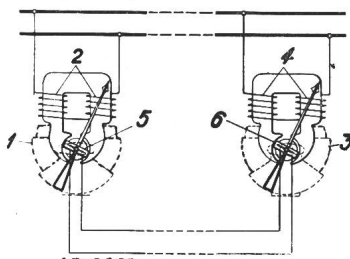
Fig. 1. Grundschaltung der Fernmessung. 1 und 3: Geber bzw. Empf. 2 und 4: deren Feldwicklg. 5 und 6: deren Drehspulen.
