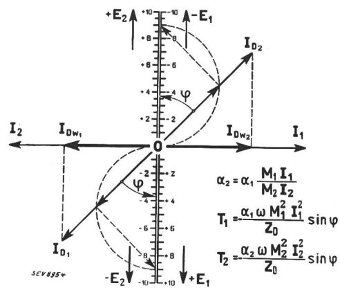
Fig. 2. Vektordiagramm zur Grundschaltung nach Fig. 1.
