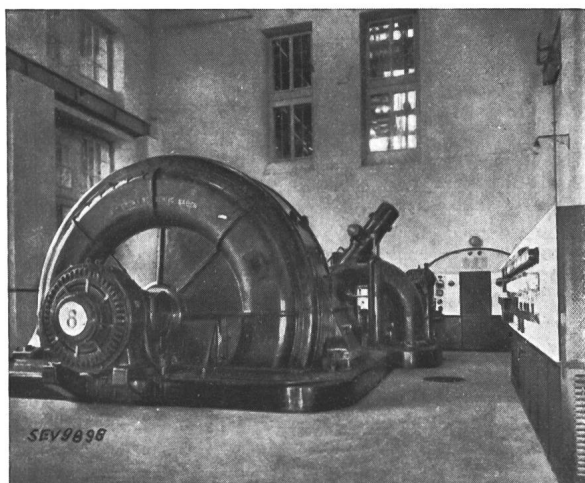
Fig. 6. Lötschwerk. 12 000-kVA-Drehstromgenerator 8.
