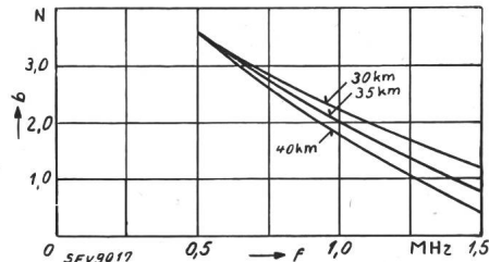
Fig. 4. Werte des Dämpfungsausgleichs für 30..40 km.
