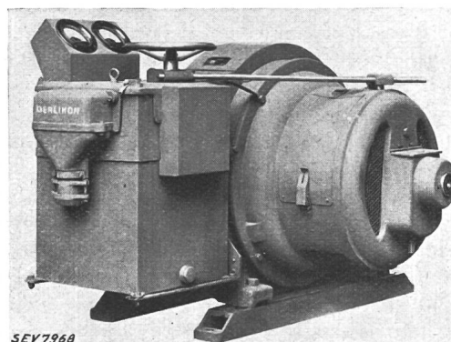
Fig. 13. Drehstrommotor mit angebautem Anlassapparat mit Statorschalter und verriegelt mit der Kurzschluss- und Bürstenabhebevorrichtung.
