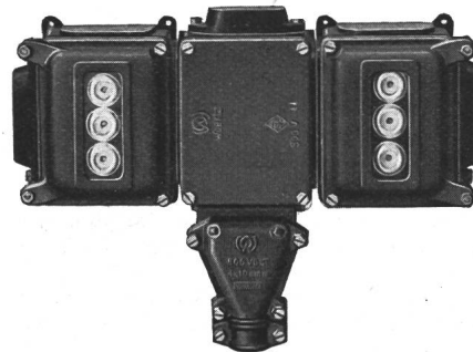
Guss-Sicherungskasten.
