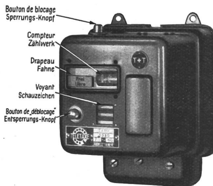
Compteurs de taxes téléphoniques «TELETAXE» de SODECO
