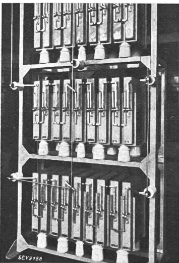
Oben: Hochspannungs-«Nepolin»-Kondensatoren-batterie von 500 kVar, 6000 V, 50 Hz.
