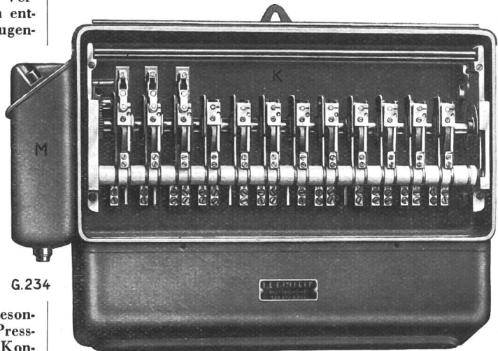
Motorantriebenes Kontaktwerk.
