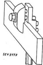
Sammelschienenklemme.
