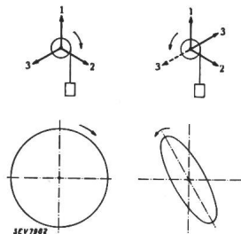
Diagramme vectoriel et champs tournants correspondants du couplage de freinage combiné hyper- et hypo-synchrone avec inversion d'une phase.
