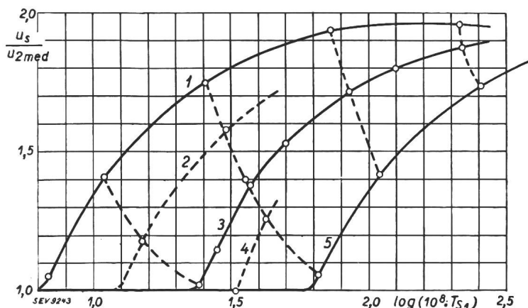
Fig. 8. Scheitelwert in Abhängigkeit von der Zeit bis zum ersten Scheitelwert. 1 24 kV/cm, 2 12 kV/cm, 3 6,7 kV/cm, 4 4,8 kV/cm, 5 2,4 kV/cm. Die Trajektorien verbinden die Punkte L \cdot C = konstant.
