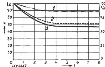
Fig. 1. Diminution de l'éclairage (E) en lux après nettoyage pour des appareils de types divers. t Temps en semaines. 1 Diffuseur fermé. 2 Coupe pour éclairage semi-indirect. 3 Coupe pour éclairage indirect.
