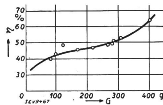
Fig. 3. Zusammenhang zwischen der Stromausbeute \eta in % und dem Elektrodenvorschub G in Gramm.
