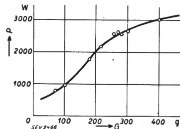
Fig. 2. Zusammenhang zwischen der elektrischen Leistung P in Watt und dem Elektrodenvorschub G in Gramm.
