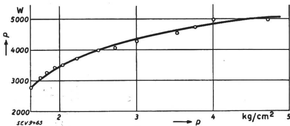
Fig. 1. Zusammenhang zwischen der elektrischen Leistung P in Watt und dem Druck des Belastungsstromes p in \text{kg/cm}^2 .
