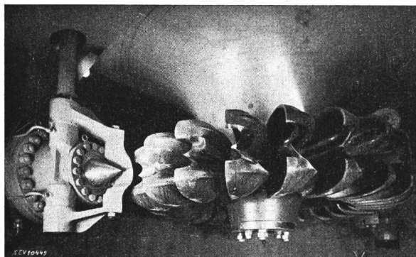
Fig. 12. Turbinenlaufrad mit Düsenadel und Strahlablenker (Escher-Wyss).
