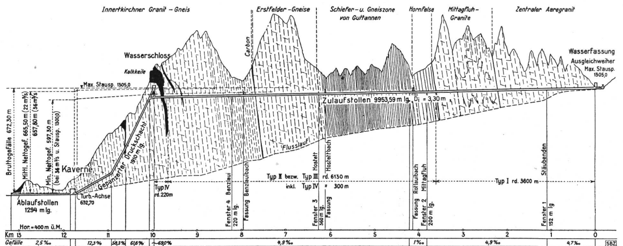
Fig. 3. (Aus Schweiz. Bauztg., Bd. 120 (1942), Nr. 3) Geologisches Längenprofil der unteren Kraftwerkstufe
