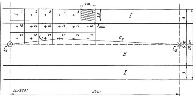
Fig. 18. Situationsplan der Strasse mit Punkteinteilung für die Berechnung der Bodenbeleuchtungsstärken. I Trottoir. II Fahrbahn.
