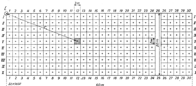
Fig. 19. Flächeneinteilung für die Berechnung des Boden-Beleuchtungswirkungsgrades.
