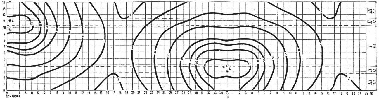
Fig. 3. Horizontalbeleuchtungsstärken auf der Bodenfläche. Isoluxkurven (int. Lux) zwischen zwei Lichtpunkten. L Lampe, I Fahrbahn, II Fahrradweg, III Trottoir.
