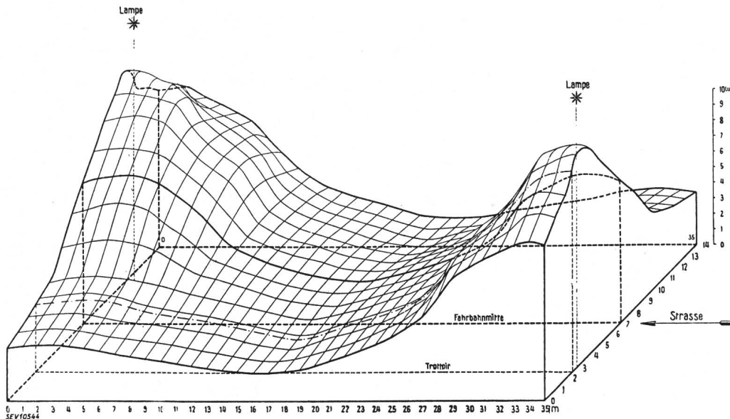
Fig. 4. Horizontalbeleuchtungsstärken auf der Bodenfläche in int. Lux zwischen zwei Lichtpunkten.
