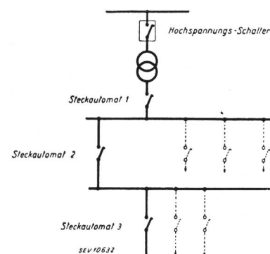
Fig. 1. Schema einer Verteilanlage
