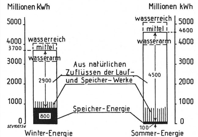
Fig. 3. Mögliche Gesamtenergie aller Wasserkraftwerke Stand 1942
