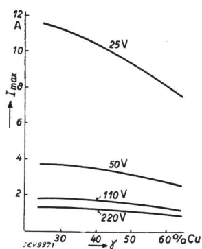
Fig. 6. Grenzstromstärken ( I_{max} ) für Wolfram-Silber-Verbundmetalle in Abhängigkeit von der elektrischen Leitfähigkeit ( \gamma in % Cu).
