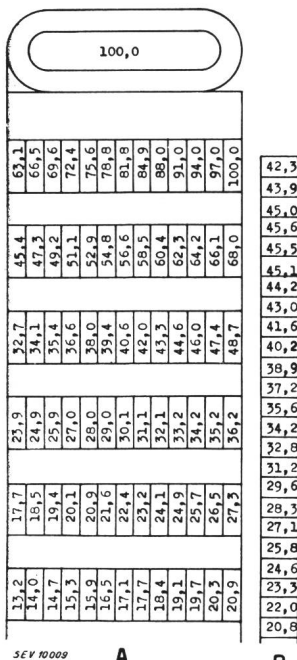
Fig. 13. Ohne Spulenverbindungen.
