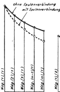
Fig. 9. Spannungverteilung über der 1. Halbspule.
