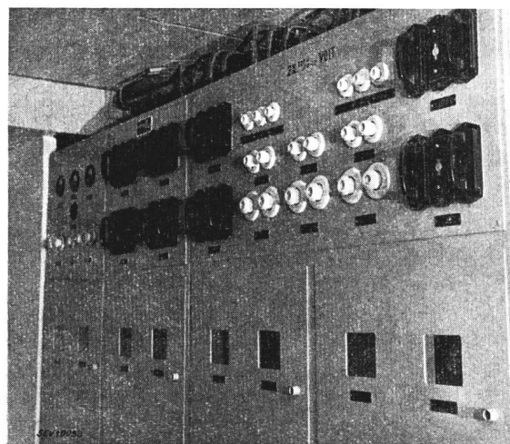
Fig. 1. Hauptverteiltafel I: Beleuchtung 440/220 V.
