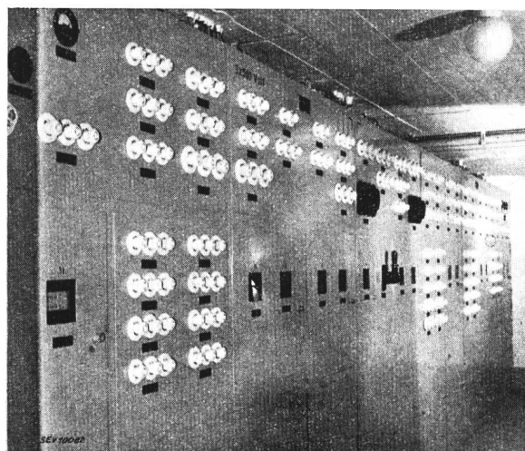
Fig. 2. Hauptverteiltafel II: Drehstrom 3 × 500 V, Drehstrom 3 × 380/220 V.
