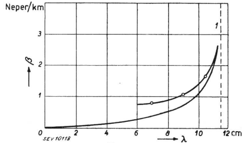
Fig. 3. Gemessener und errechneter Frequenzgang der Dämpfung bei quadratischer Gleichrichtung. \lambda Wellenlänge (1 Grenzwellenlänge), \beta Dämpfung.
