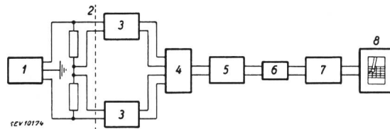
Fig. 2. Anordnung für Untersuchungen über hochfrequente Gleichlauf-Steuerung.
