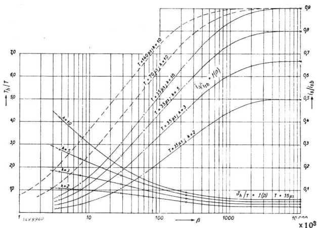
Fig. 11. Kurvendarstellungen
