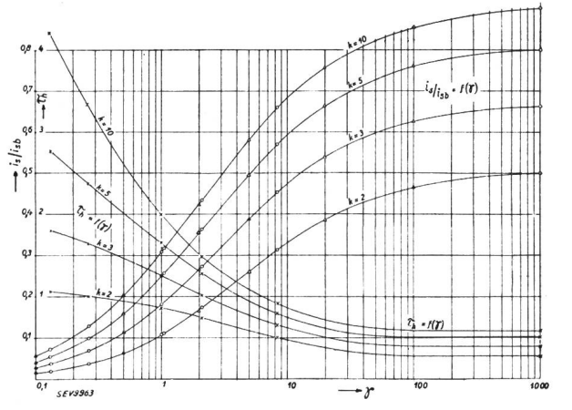
Fig. 14. Kurvendarstellungen
