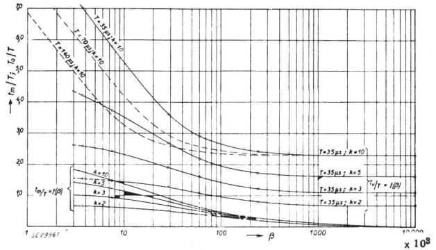
Fig. 12. Kurvendarstellungen
