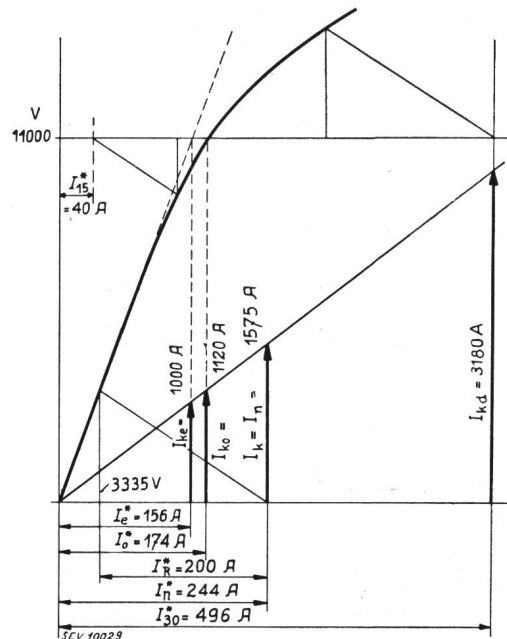
Fig. 18. Résultats d'essais en usines. Caractéristiques à vide et en court-circuit; triangle de Potier.
