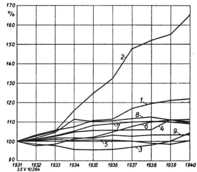
Fig. 3. Entwicklung des mittleren Anschluss- wertes pro Apparat 1931...1940 (1931 = 100).
