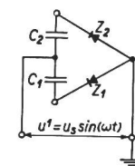
Fig. 4b. Verdopplungsschaltung
