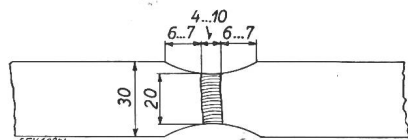
Fig. 2. Zugprobe
