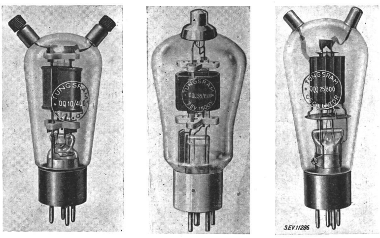
Fig. 3. Spezial-UHF-Senderöhren Tungsram OQ 10/400, OQQ 55/1500, OQQ 25/800 mit 10, 55, 25 W Anodenverlustleistung (ca. 1/4 nat. Grösse).
