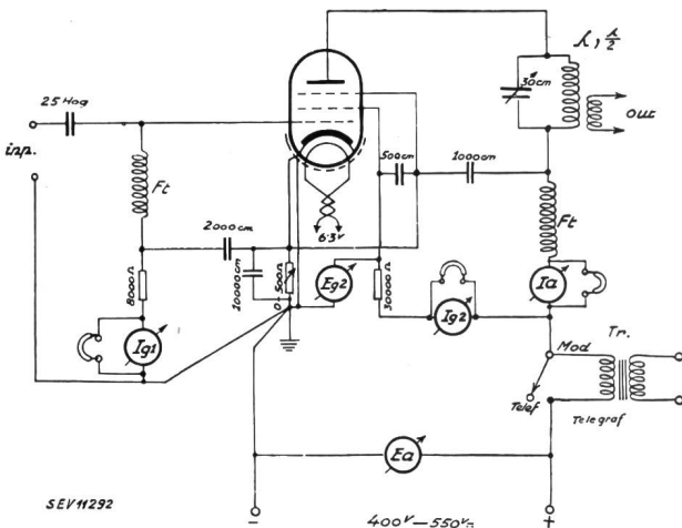
Fig. 9. 5-m-Sender mit Pentode (mit Frequenzverdoppelung)
