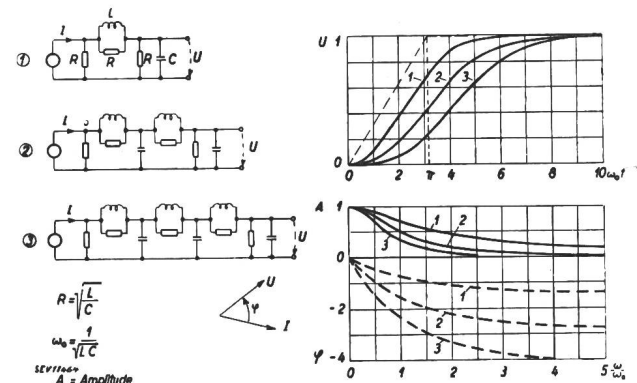
Fig. 14. Sprung und Tiefpass
