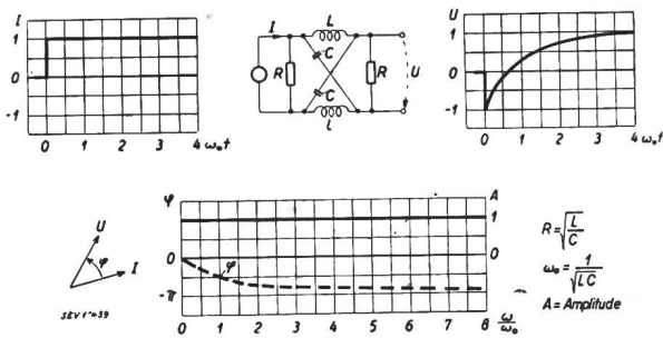
Fig. 9. Einheitssprung und Kreuzglied
