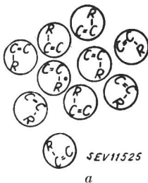
a Schema von Mikromolekülen einer polymerisier- oder kondensierbaren Flüssigkeit. Gleichwertigkeit aller Nachbarn.
