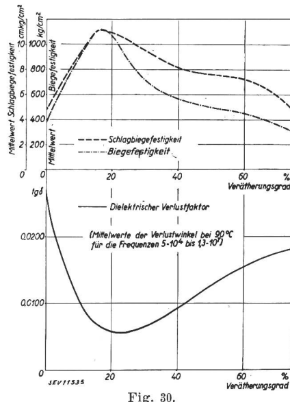
Fig. 30. Mechanischen Eigenschaften und dielektrischer Verlustfaktor verschiedener Phenolabkömmlinge
