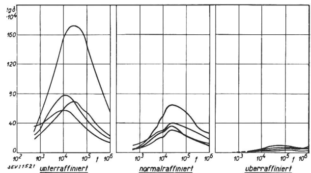
Fig. 16. Abhängigkeit des dielektrischen Verlustfaktors vom Raffinationszustand (Gemeinschaftsversuche J.E.C.)
