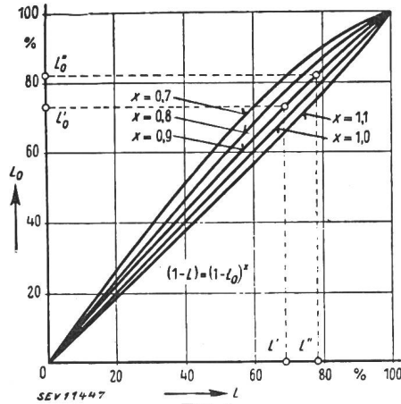
Fig. 4. Courbes d'étalonnage
