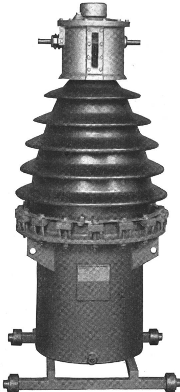
Fig. 1. Stützstromwandler für Aussenbetrieb 65 kV Nennspannung, 152 kV Prüfspannung, 120...240 A, 70 VA, Klasse 0,5 + 200 VA, Klasse 1,0 50 Hz.
