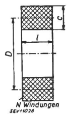
Fig. 1. Querschnitt durch die Spulenachse D mittlerer Durchmesser. l Spulenlänge. c Spulendicke.
