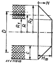
Fig. 3. Feld der unendlichlangen Spule
